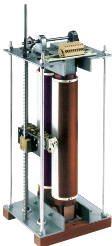
Einphasiger Säulenstelltransformator
