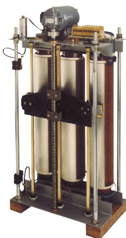
Dreiphasiger Säulenstelltransformator
