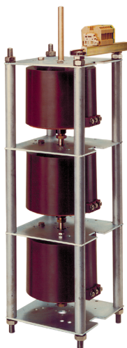
Dreiphasiger Ringstelltransformator
