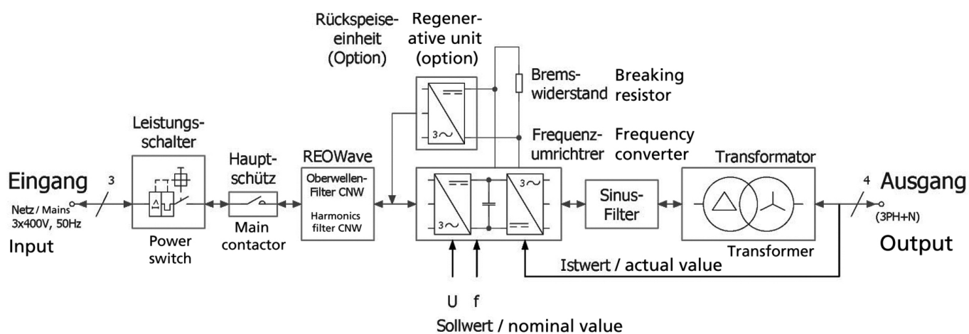
Blockschaltbild
