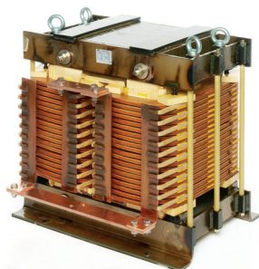
Einphasen-Lastdrossel NPT
